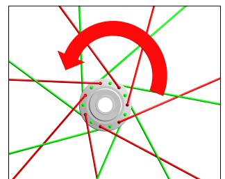
ROUES AVANT CÔTÉ OPPOSÉ À LA TRANSMISSION
