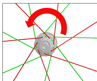
HINTERRAD NICHTANTRIEBSSEITE
